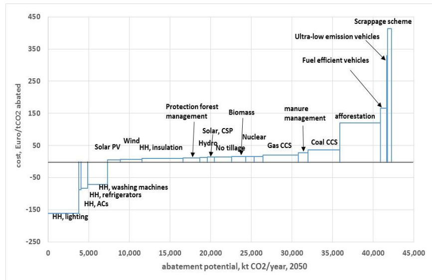
Figura 1: Curba costurilor marginale de reducere a emisiilor, la nivel transsectorial, 2050
